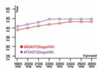
RX serie vermogen vergelijking (Stage IIIA/IIIB)
