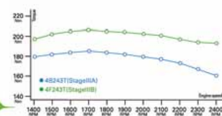
RX Serie Koppel vergelijking (Stage IIIA/IIIB)
